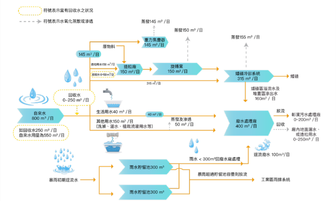
鋼聯用水平衡圖
